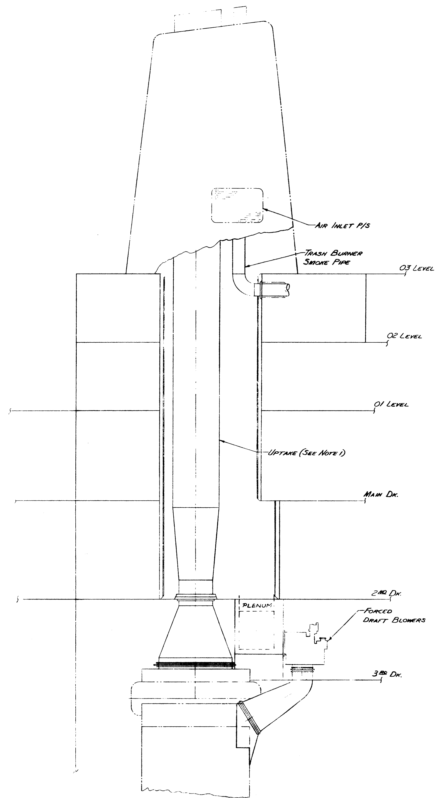
ELEVATION
